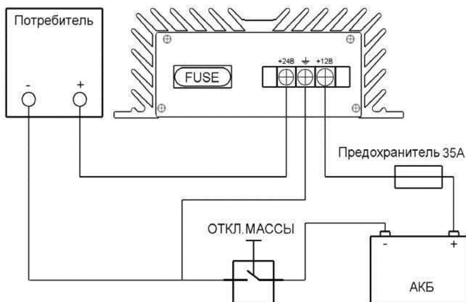
Рис. 1: Схема подключения устройства
