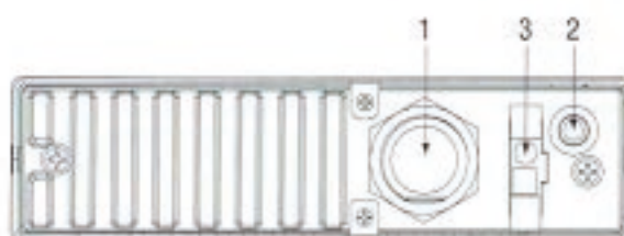
Рис. 3. Описание разъемов на задней панели радиостанции MegaJet MJ-500
